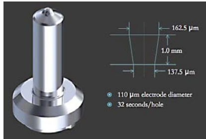
역 테이퍼 구멍
